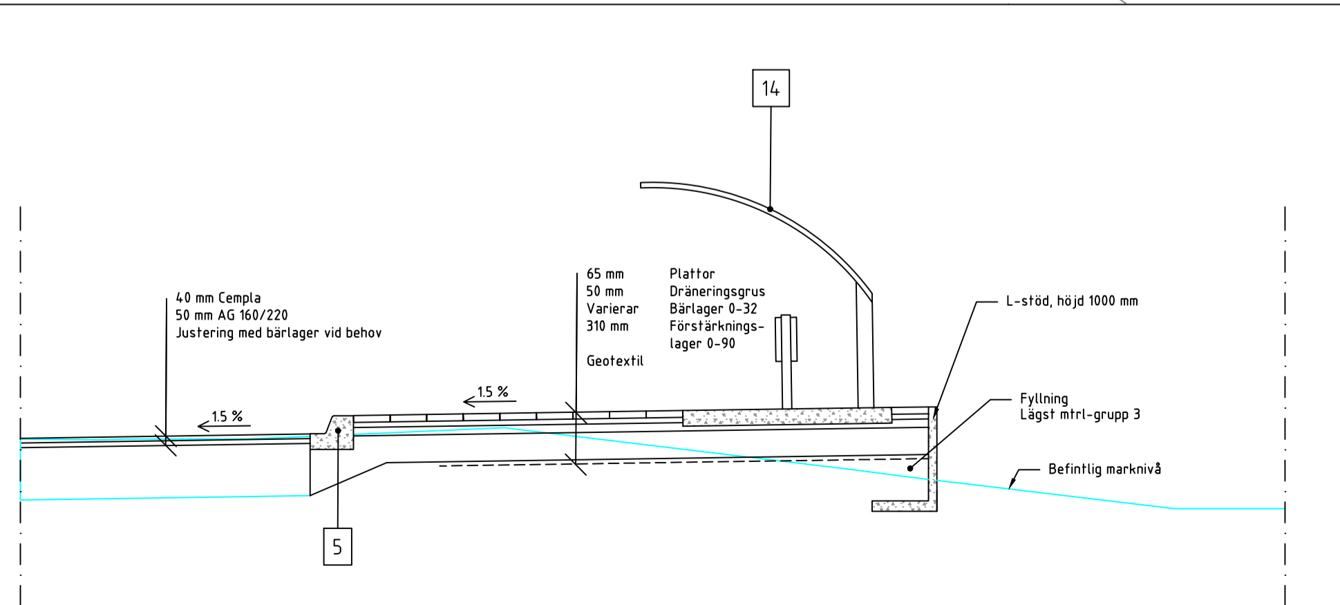
SEKTION A-A Skala 1:50
