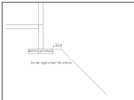
Principskiss vid schakt intill befintlig grundläggning (WSP 2023-12-12)
