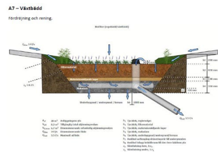
Figur 3. Sektion för växtbädd som använts i beräkningar.
