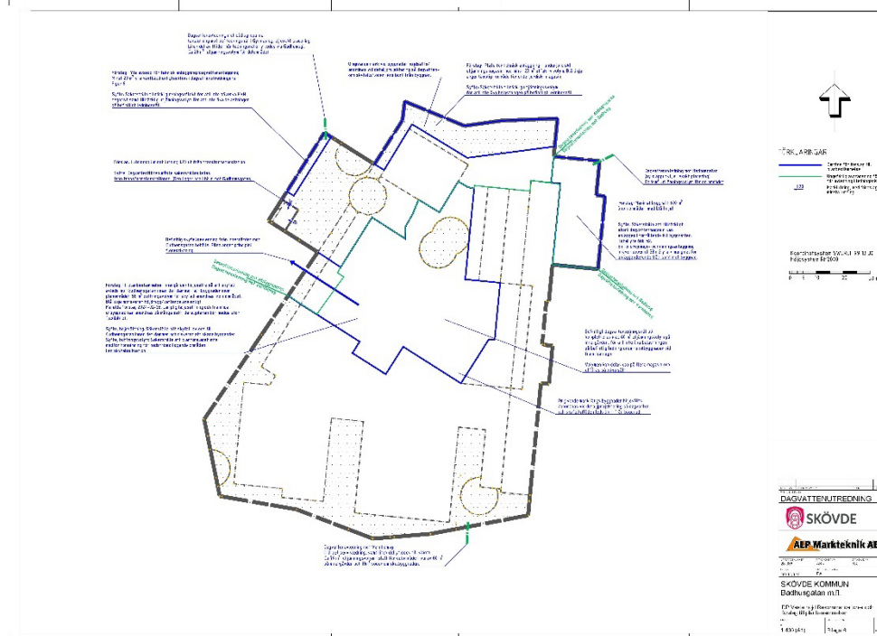
Förslag på hantering av dagvatten och skyfall är redovisat samlat på ovanstående karta. Finns i större format som bilaga 6 i Dagvatten- och skyfallsutredningen av ALP Markteknik
